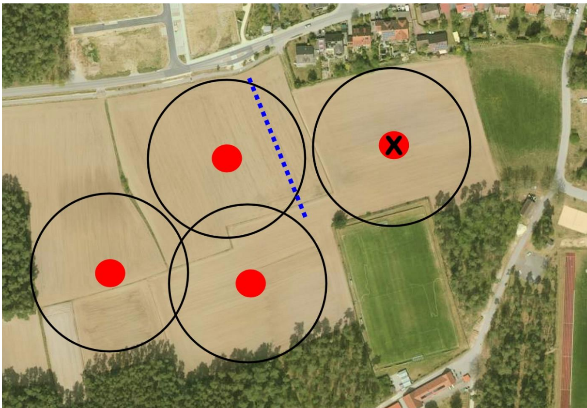
Abb. 10: Schematische Darstellung der Betroffenheit der Feldlerche gemäß "Worst-Case-Szenario". Rote Punkte: Mögliche Revierzentren der Brutpaare. Schwarze Kreise: die Radien von ca. 60 m (Durchmesser 120 m) demonstrieren die Abstände zu Vertikalstrukturen und der - leicht überlappenden - Brutreviere zueinander. Roter Punkt mit x: verloren gehendes Revier. Blaue Punktlinie: Westgrenze des Wirkungsbereiches des Vorhabens auf Feldbrüter.
