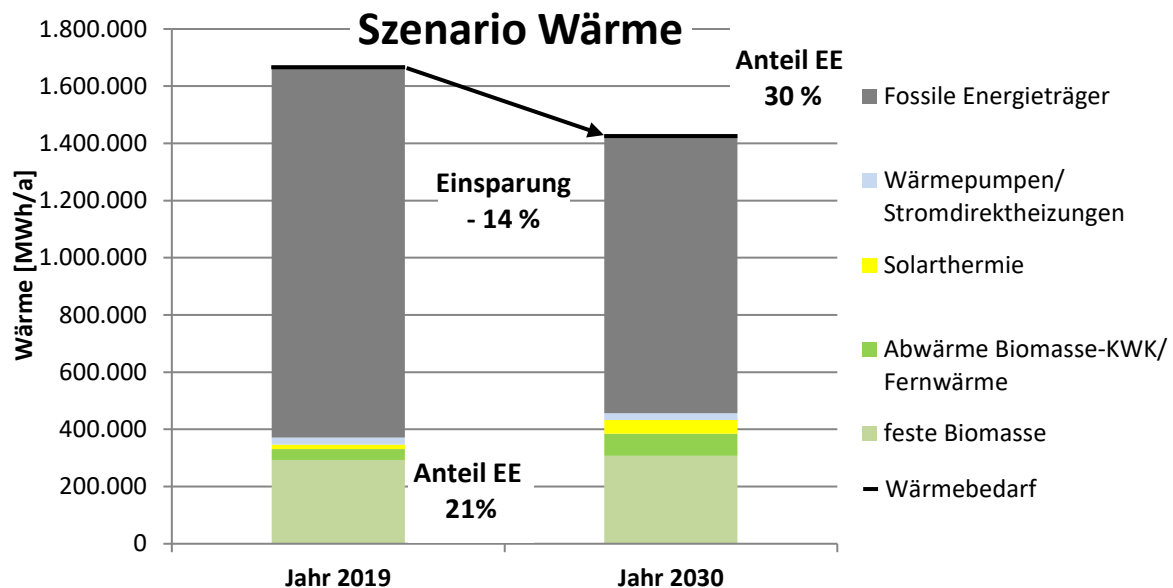
Abbildung 40: Zusammenfassung des Szenarios 2030 – Thermische Energie
