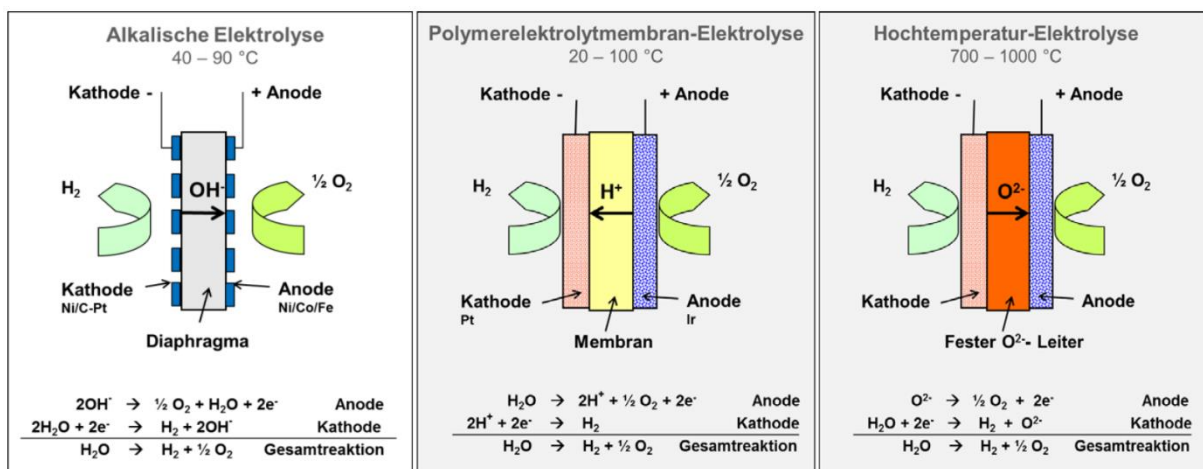
Abbildung 27: Chemische Reaktionen verschiedener Elektrolyse-Arten [DLR]
