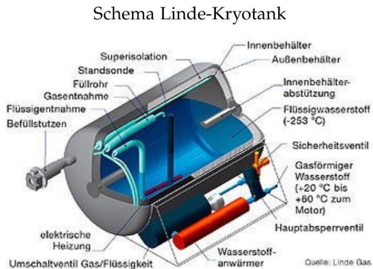
Abbildung 30: Speicherung von verflüssigtem LH 2 in speziellen Tanks [Fraunhofer ISE]
