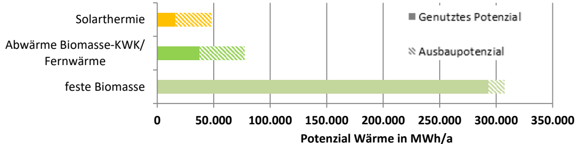
Abbildung 17: Genutzte Potenziale und Ausbaupotenziale erneuerbarer Energien zur Wärmeerzeugung
