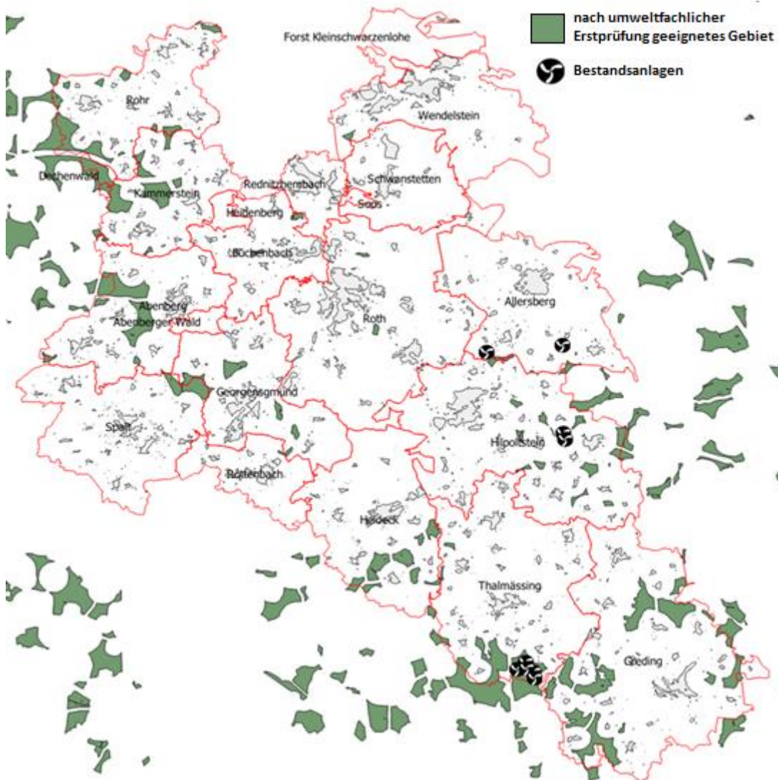
Abbildung 21: Studien des Öko-Instituts Bayern zufolge nach umweltfachlicher Erstprüfung geeignete Gebiete für Windkraftanlagen ([LfU Wind], eigene Bearbeitung)
