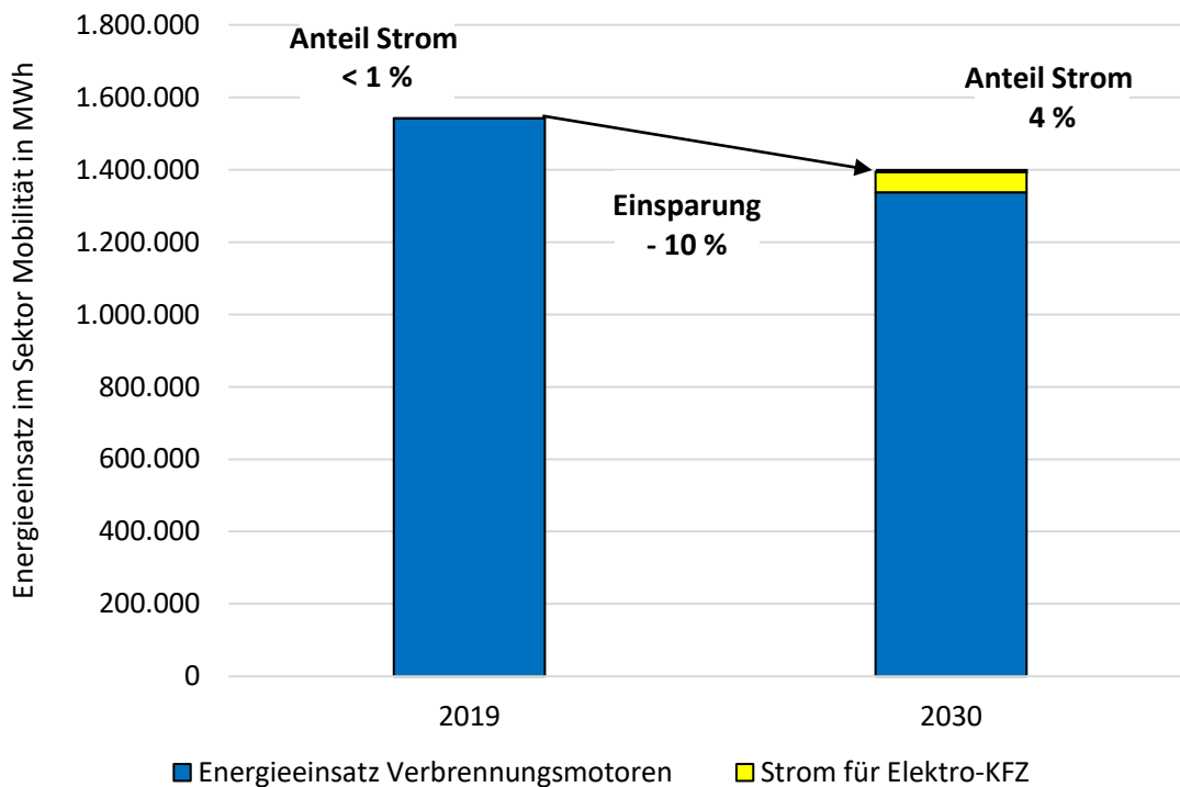
Abbildung 41: Zusammenfassung des Szenarios 2030 – Verkehr
