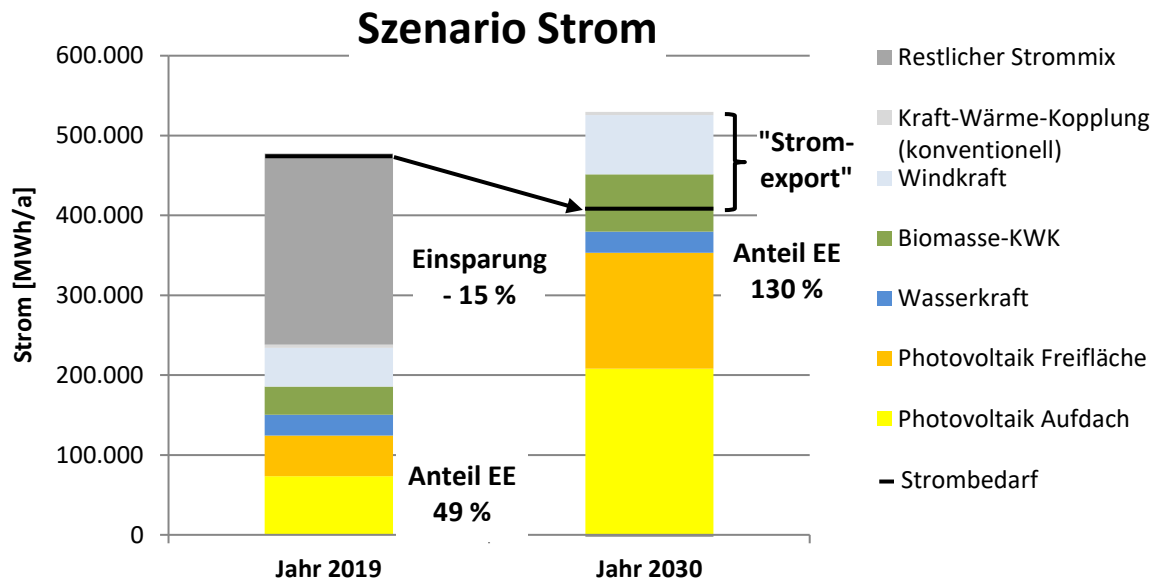
Abbildung 39: Zusammenfassung des Szenarios 2030 – Strom
