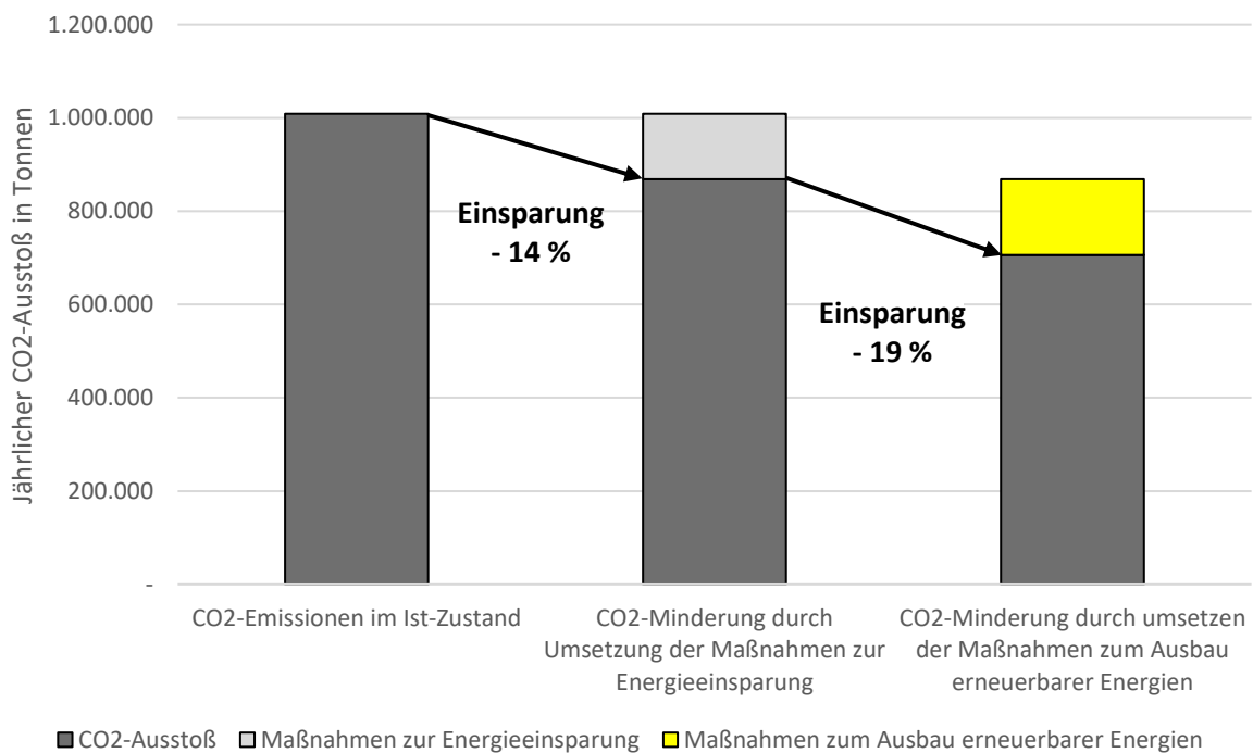
Abbildung 25: Entwicklung der CO 2 -Emissionen
