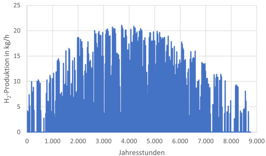
Abbildung 36: Potenzielle Wasserstoff-Produktion mit PV-Strom an der Deponie Pyras
