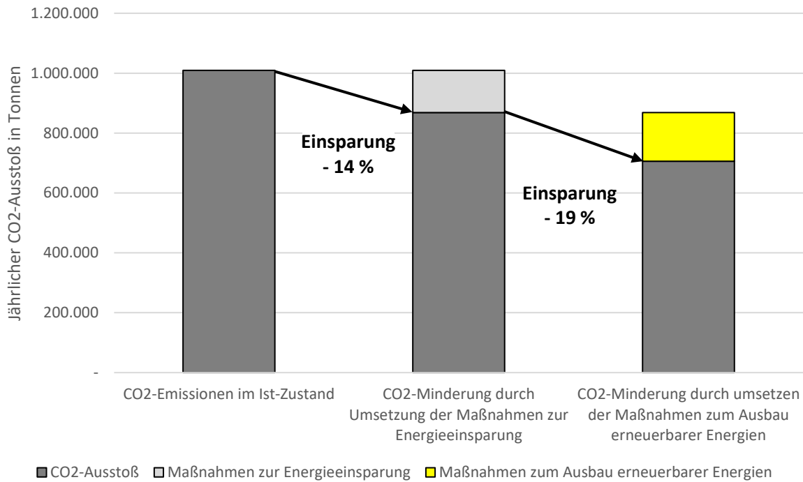
Abbildung 42: Zusammenfassung des Szenarios 2030 - Entwicklung der CO 2 -Emissionen
