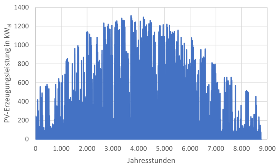
Abbildung 35: Erzeugungzeitreihe einer 1,6 MWp-PV-Anlage auf der Deponie Pyras
