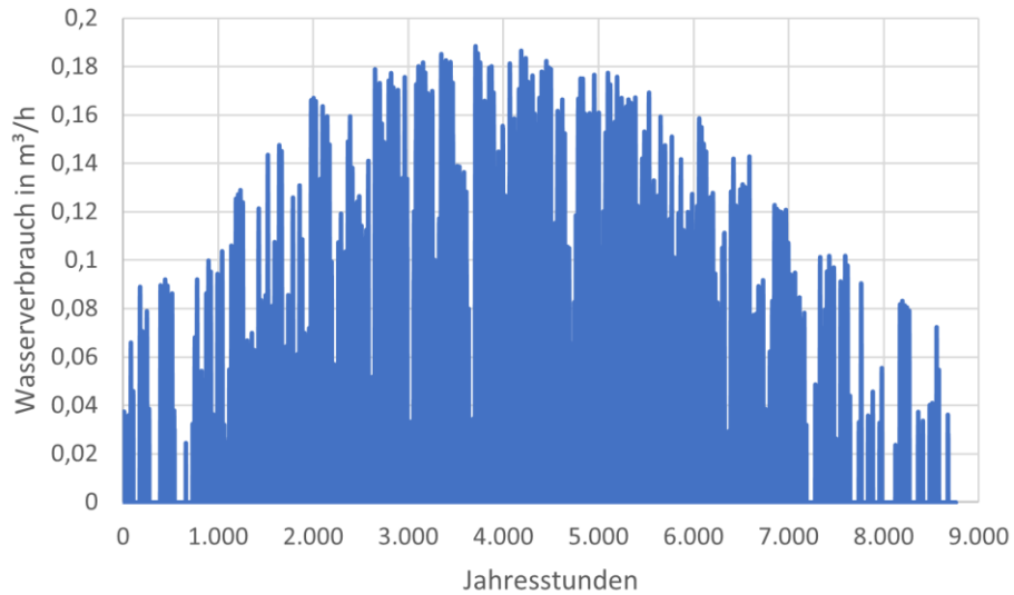
Abbildung 34: Wasser-Bedarf des Elektrolyseurs
