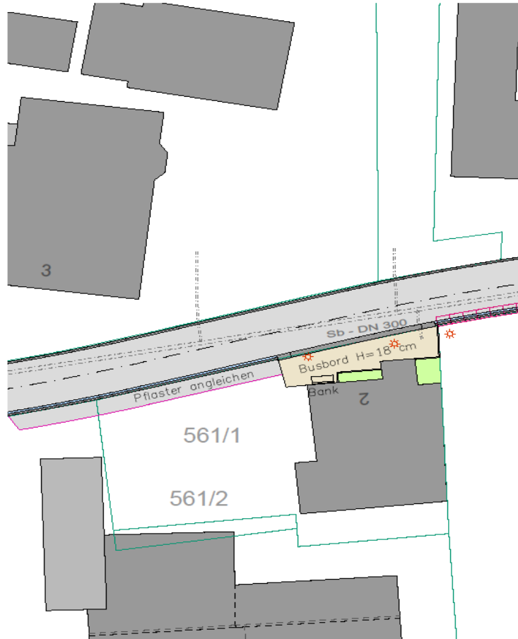
Büchenbach OT Götzenreuth – Ausbau der Lindenstraße und Buchenstraße Detail Bushaltestelle Lindenstraße M 1:200 29.08.2023
